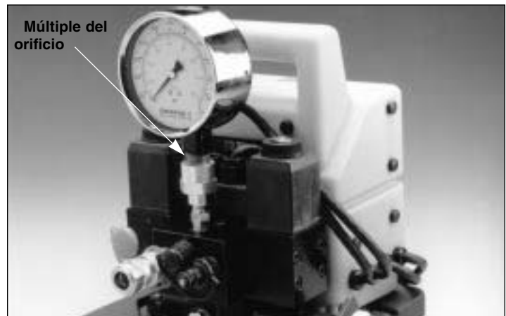
Figura 3, Múltiple del orificio de la bomba
